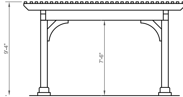
End Elevation
