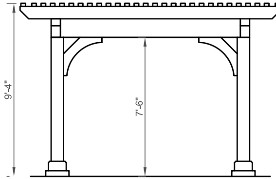
End Elevation
