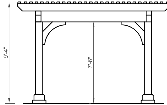
End Elevation
