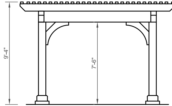
End Elevation
