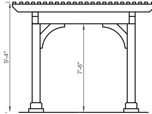
End Elevation
