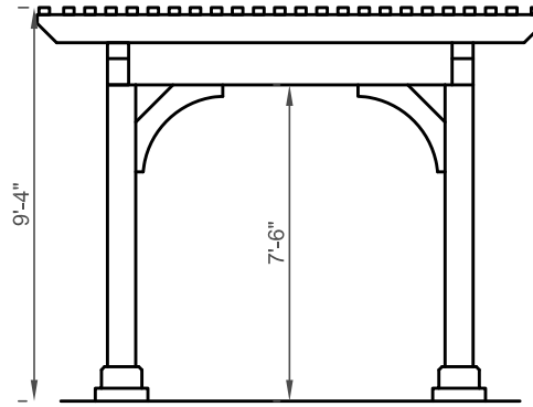
End Elevation
