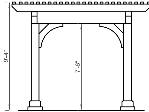
End Elevation
