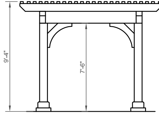
End Elevation
