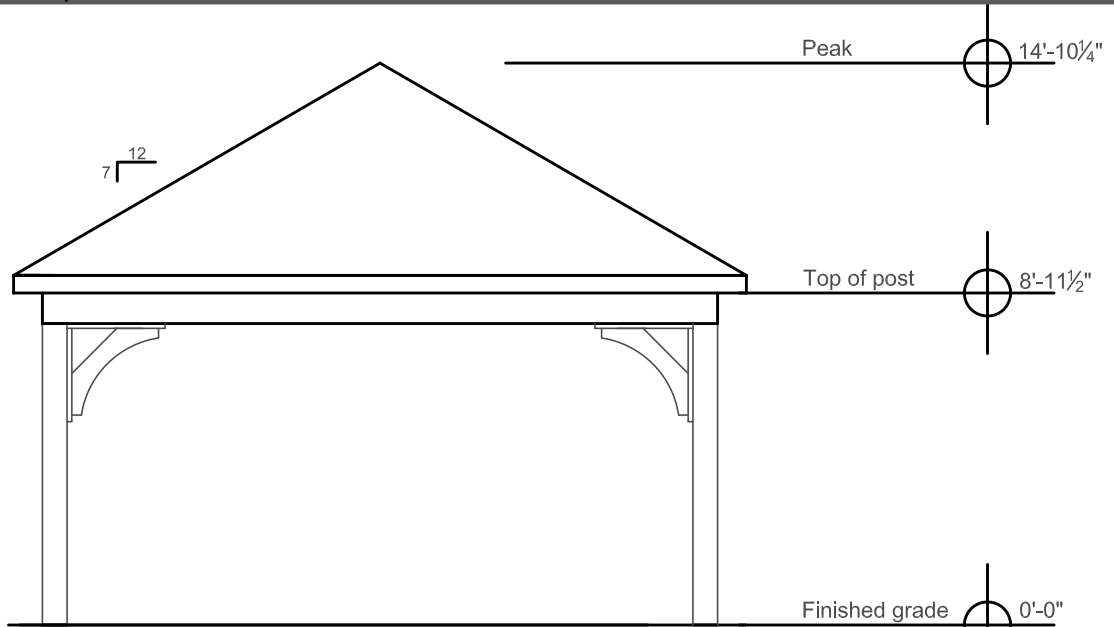
End Elevation
