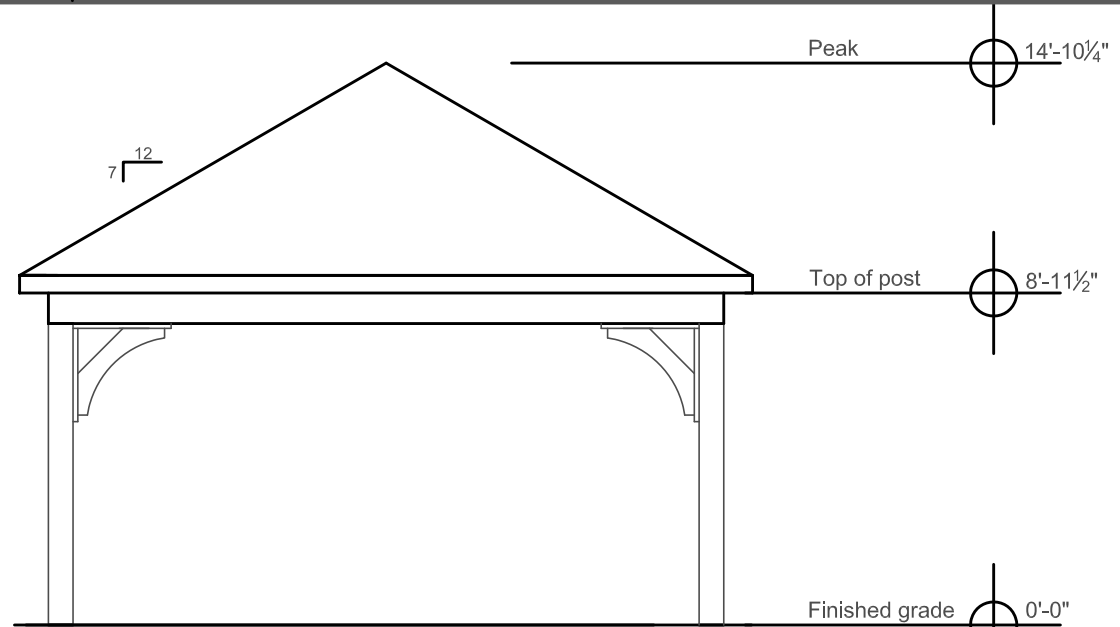
End Elevation
