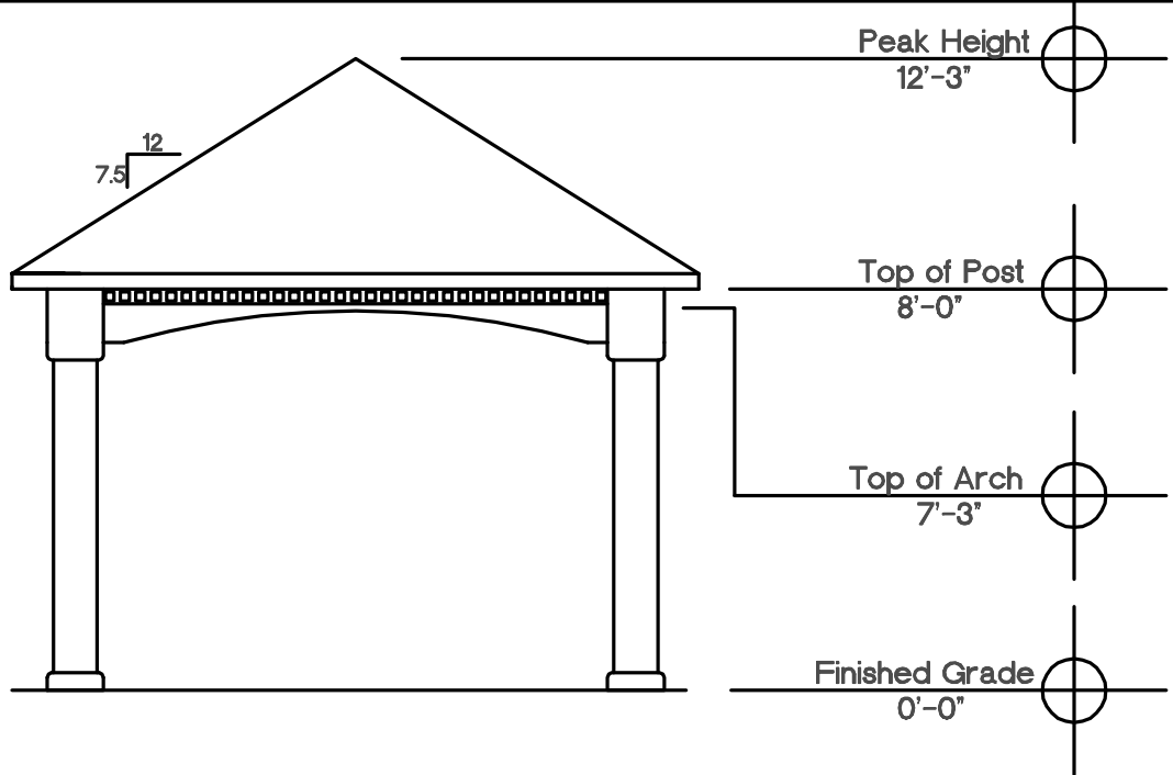
End Elevation 12'x14'
