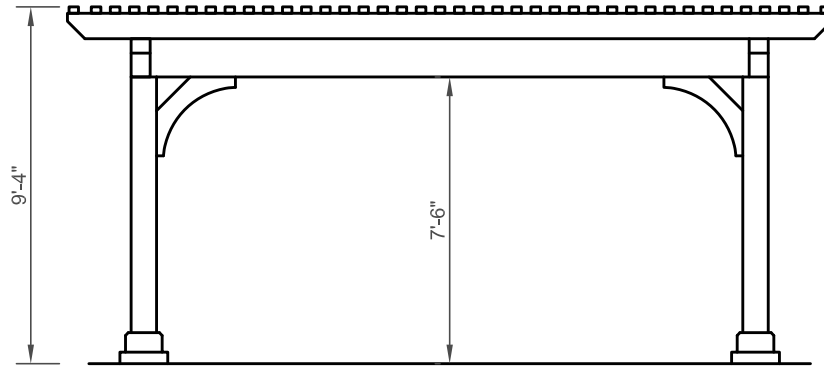
End Elevation
