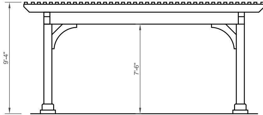
End Elevation
