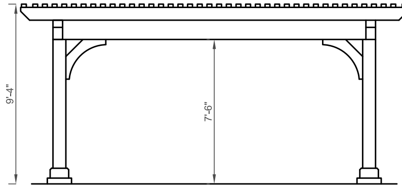
End Elevation
