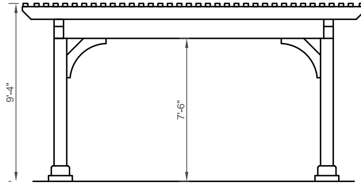
End Elevation
